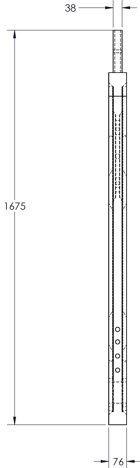
VISTA LATERAL ESC: 1:10
