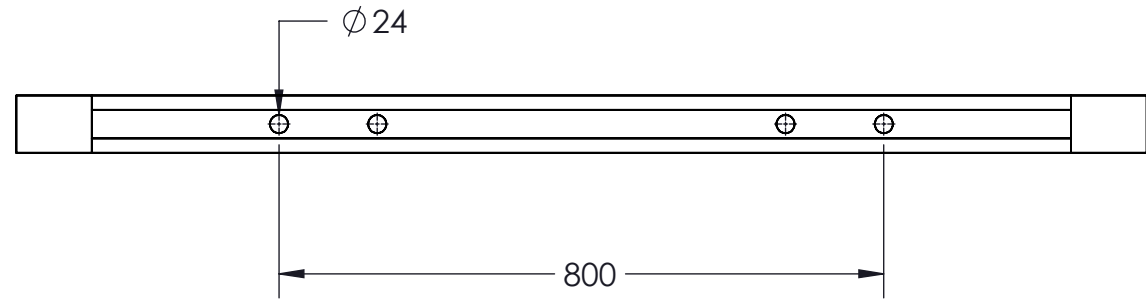
VISTA SUPERIOR ESC: 1:10
