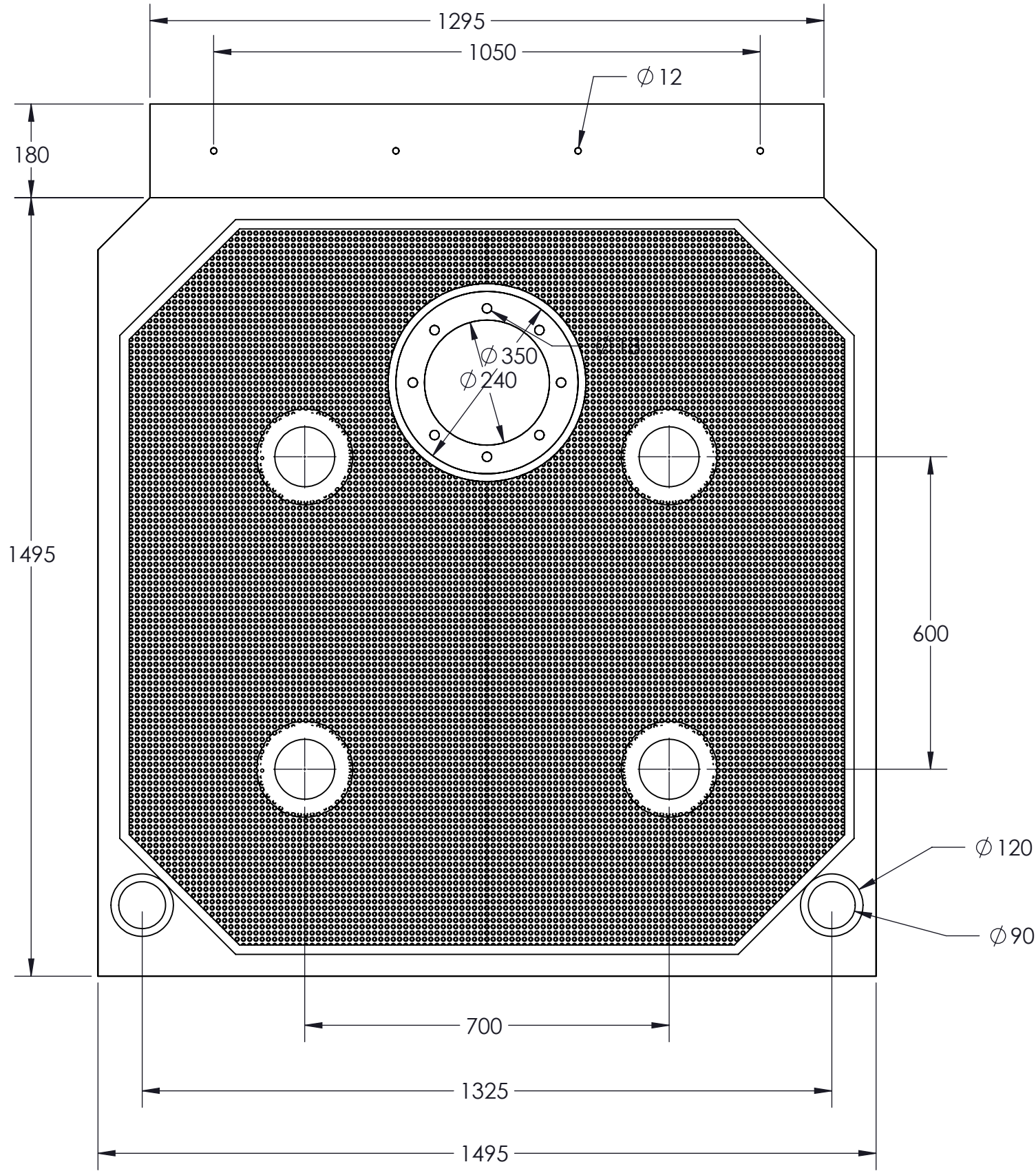
VISTA ELEVACION ESC: 1:10
